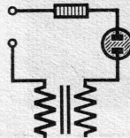
Links: Abb. 1. Unterfuchung der Isolation, die zwischen den 2 Wicklungen eines Niederfrequenz-Transformators vorhanden sein soll. Ist die Isolation in Ordnung, so bleibt die Glühlampe dunkel. Ebenso prüfen wir die Isolationen der beiden Wicklungen gegen den Eisenkern.
